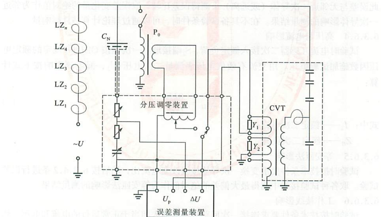
图7 用电容分压器检验电容式电压互感器的线路
