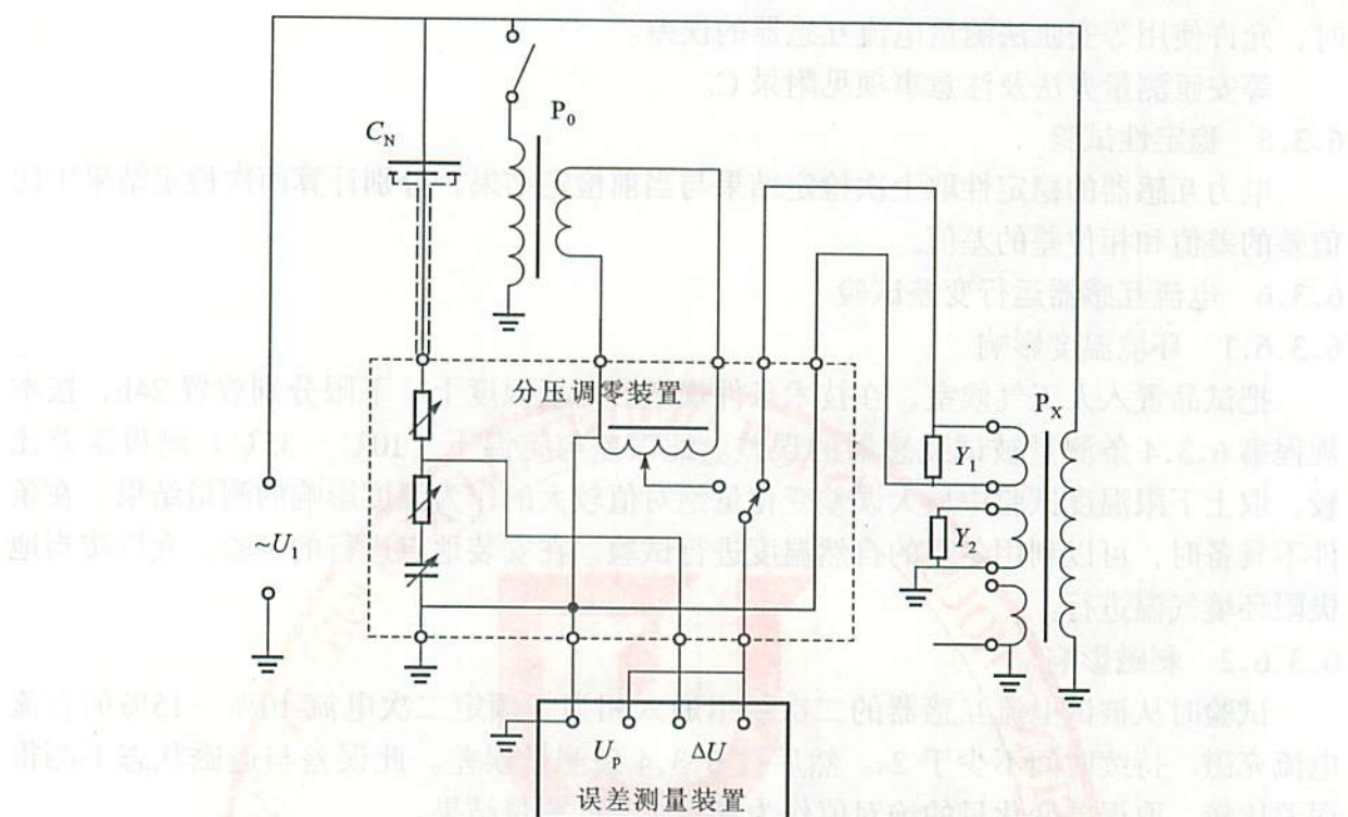
图6 用电容分压器检验电磁式电压互感器的线路
